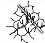
R. sachalinensis
